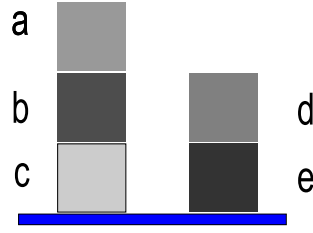
Figura 1: Definición de Sobre(x) y SoMe(x)
